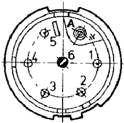
Plug (Front View) Stecker (Vorderansicht)
